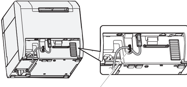
Kablo kancası: kablonun düşmesini önler.
